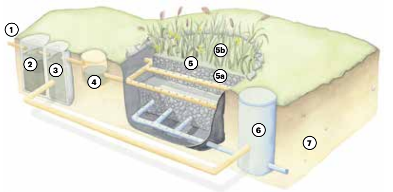
Vtok odpadne vode (1), Troprekadni usadnik (2), Dotočno črpališče (3), Doziranje obarjalnega sredstva za fosfor (4), Čistilna greda (5), pesek različne granulacije (5a), vlagoljubne rastline (5b), Iztočni jašek / črpališče za interni povratek (6), Izток čiščene vode (7)
